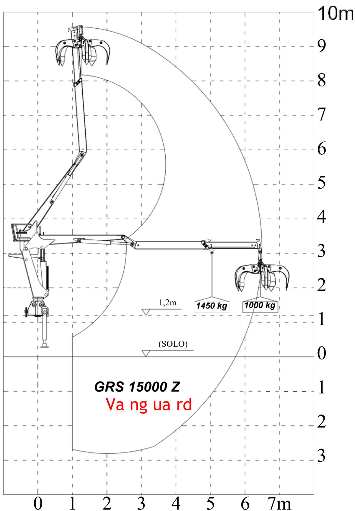
FIGURA 1 - Dimensional do guindaste.
